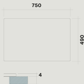
Installation semi-affleurante Schéma d'encastrement
