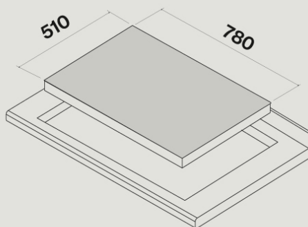
Installation semi-affleurante Schéma d'encastrement
