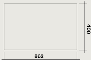
Dimensions d'encastrement, installation semi-affleurante
