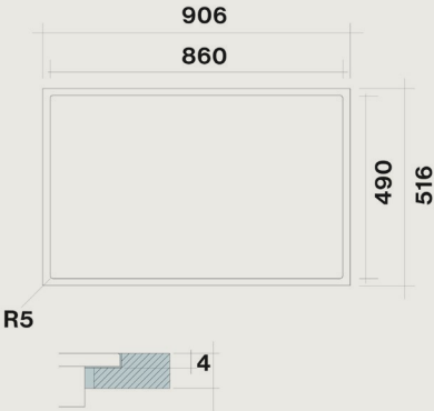
Installation à fleur Schéma d'encastrement
