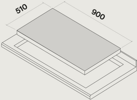
Installation semi-affleurante Schéma d'encastrement
